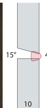
Tloušťka plechu 10 mm, faseta jednostranně 15 stupňů, vzduchová mezera 4 mm
