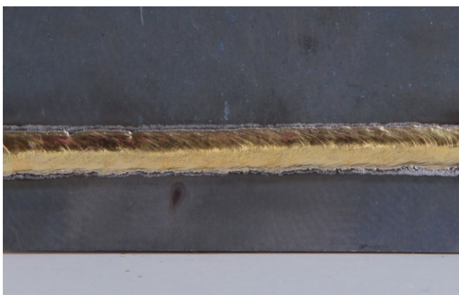
Pájení vysoce pevných plechů, např. Usibor ®
