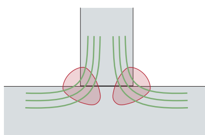
Lepší indukční tok díky hlubokému závazu
