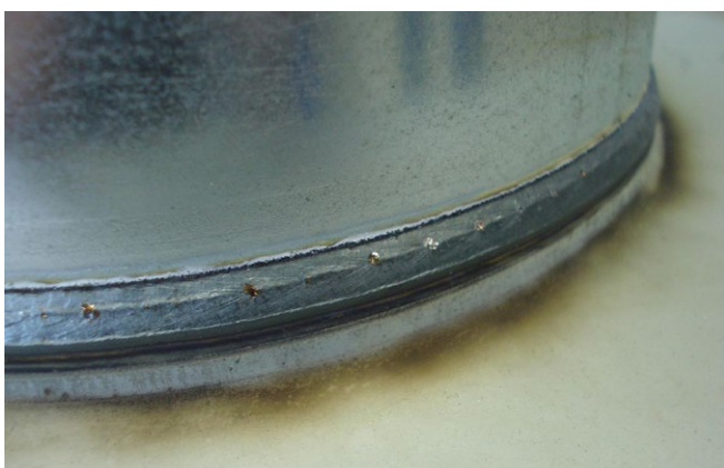
Svařování pozinkovaných plechů
