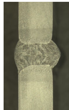
Tloušťka plechu 5 mm Vzduchová mezera 3 mm
